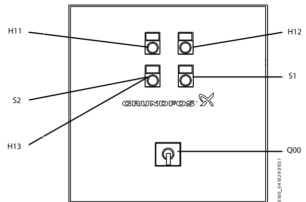
Рис. 10 Вид спереди
