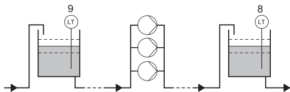
Рис. 33 Контроль уровня
