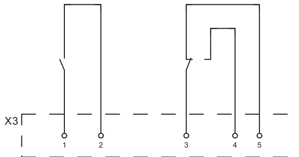
Работа мешалки
