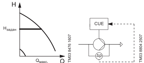
Рис. 5 Постоянный перепад давления насоса
