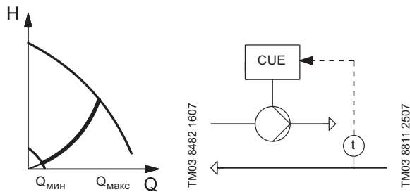
Рис. 12 Постоянная температура
