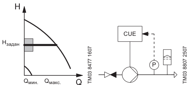
Рис. 8 Постоянное давление с функцией останова
