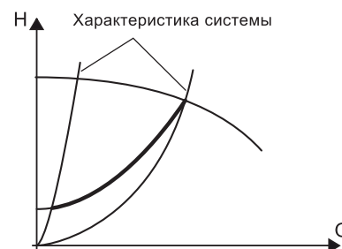
Рис. 15 Характеристика циркуляционной системы
