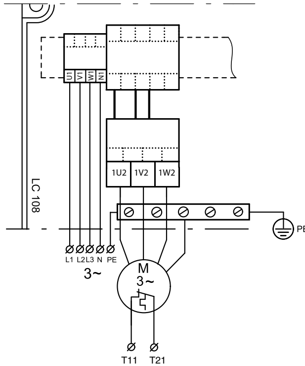
3~ DOL
