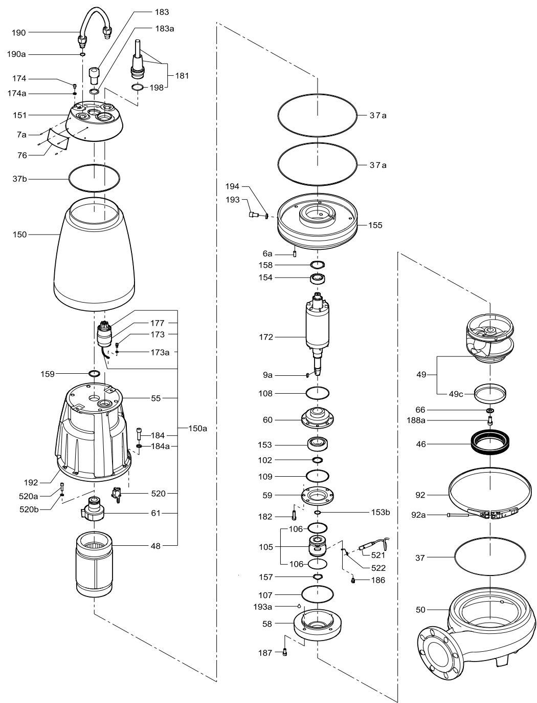
Рис. 7 Деталировка насоса SE1 с одноканальным рабочим колесом S-tube (исполнение с датчиками)
