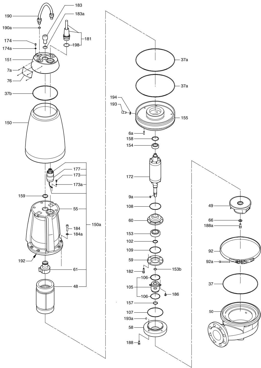
Рис. 9 Деталировка насоса SE1 со свободно-вихревым рабочим колесом типа SuperVortex
