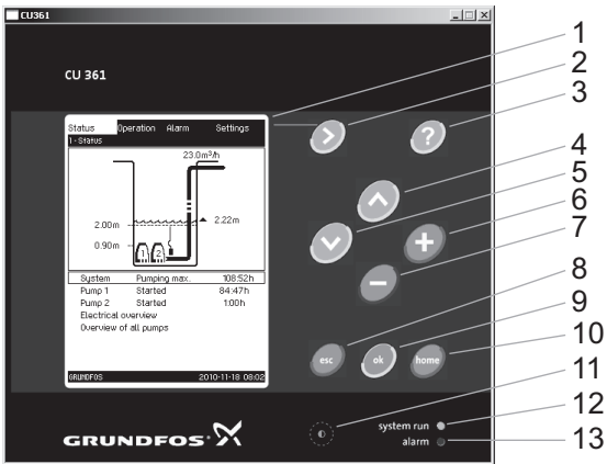
Рис. 38 Панель управления CU 361
