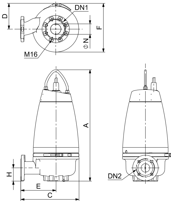
Рис. 25 Насос SEV без принадлежностей
