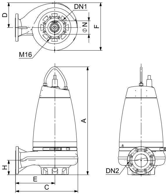
Рис. 24 Насос SE1 без принадлежностей (DN 100/DN 150)
