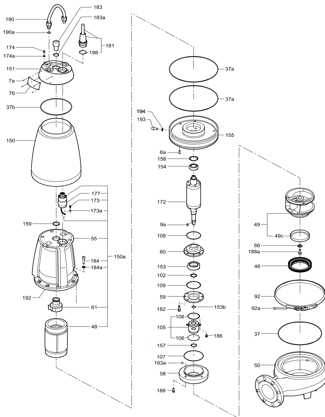
Рис. 5 Детализировка насоса SE1 с одноканальным рабочим колесом типа S-tube
