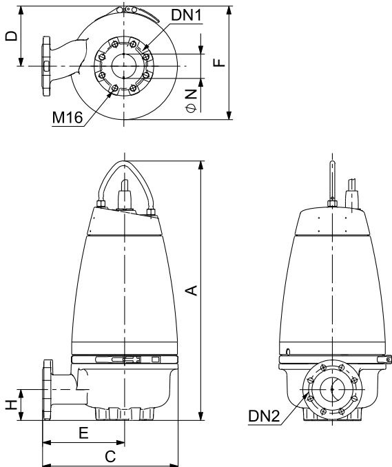
Рис. 26 Насос SEV без принадлежностей
